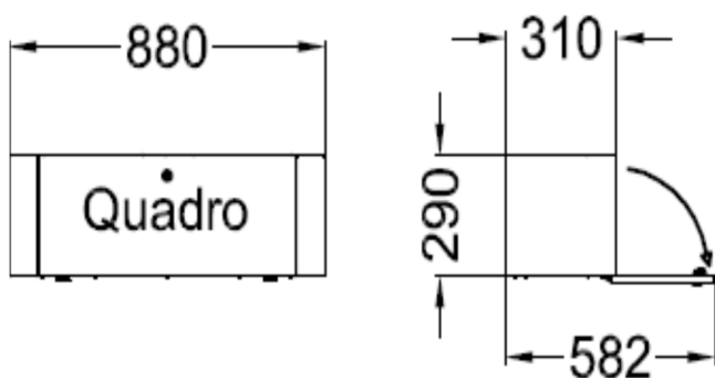
Dimensioni Quadro Manovra
